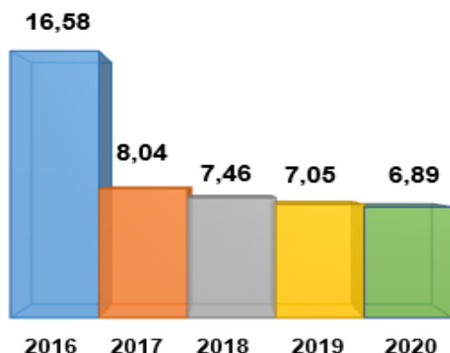
Grafic 20 – Evoluție dividend pe acțiune (lei/acțiune) în perioada 2016 – 2020
