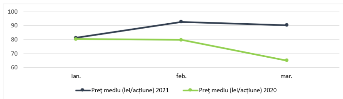
Grafic 17 - Evoluția prețului mediu de tranzacționare a acțiunilor
