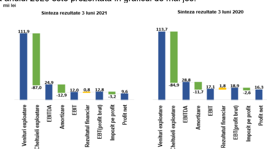
Grafic 16 - Sinteza rezultatelor financiare în perioada ianuarie-martie 2021 față de aceeași perioadă 2020
