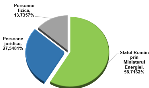
Grafic 1 - Structura Acționariatului CONPET S.A. la 31.03.2021
