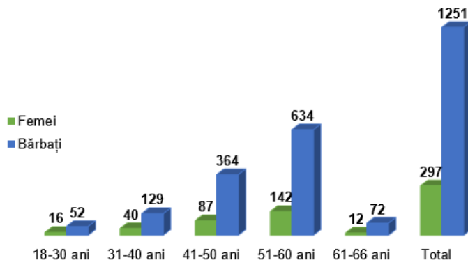
Grafic 12 - Structura personal pe gen și grupe de vârstă la 31 martie 2021
