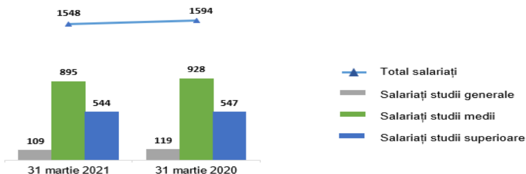
Grafic 9 – Structura salariați la 31 martie 2021 față de aceeași perioadă a anului 2020
