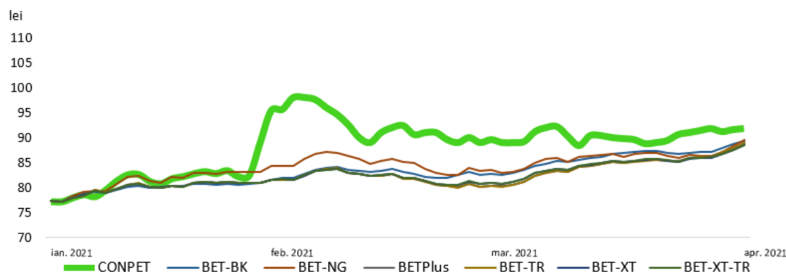
Grafic 18 - Evoluția acțiunilor COTE vs. indicele BET rebazat (lei)
