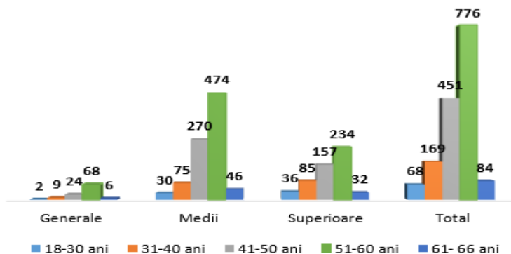
Grafic 13- Structura personal pe studii și grupe de vârstă la 31 martie 2021
