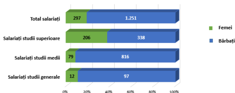
Grafic 10 - Structura personalului în funcție de gen și nivel de studii la 31 martie 2021
