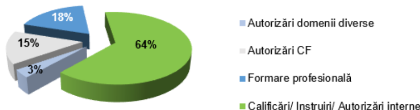
Grafic 14 – Ponderea de cursuri formare și autorizare profesională
