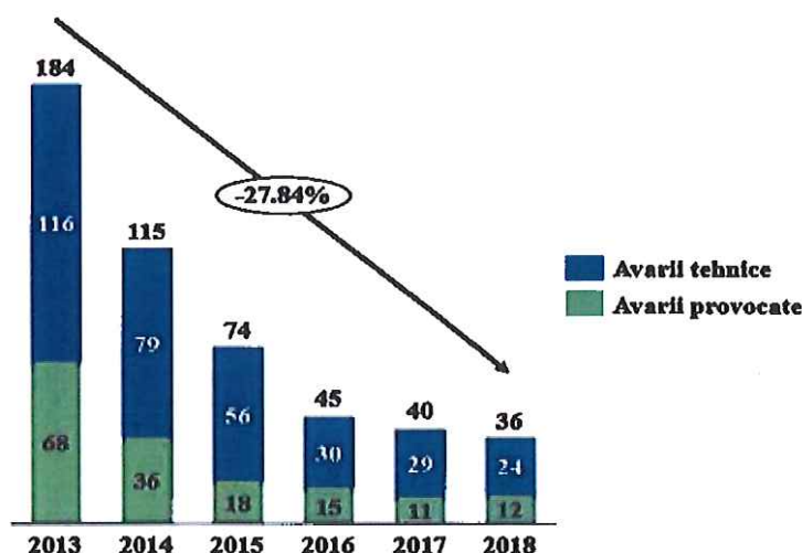
Grafic 19- Evoluția avariilor tehnice și provocate în perioada 2013-2018
