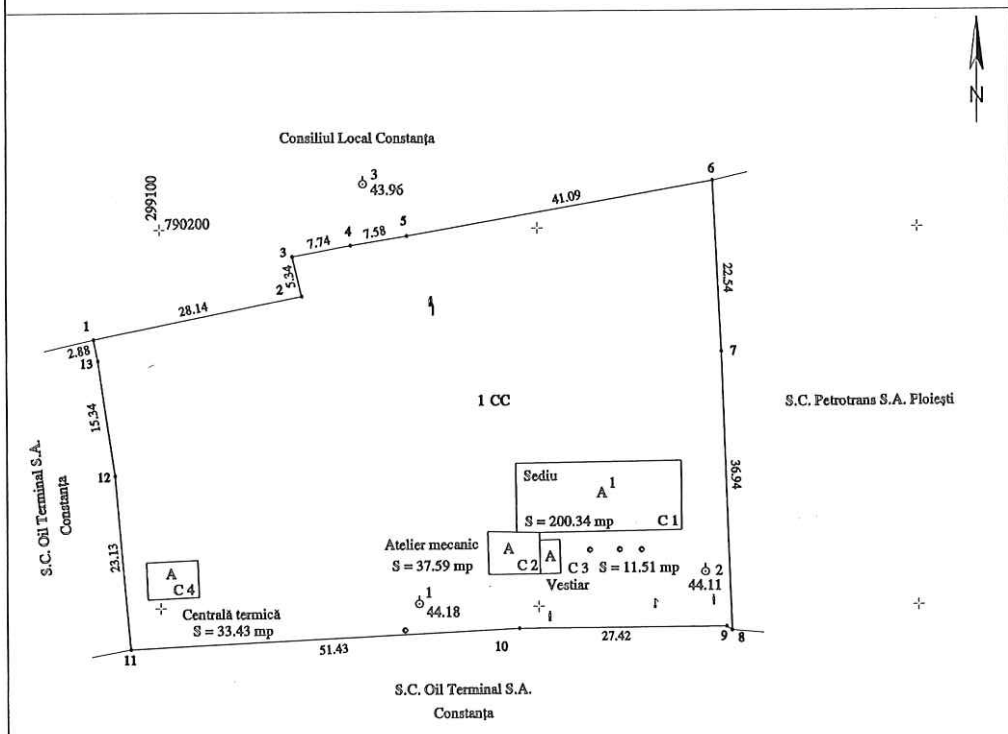
Inventar de coordonate al punctelor pe contur
